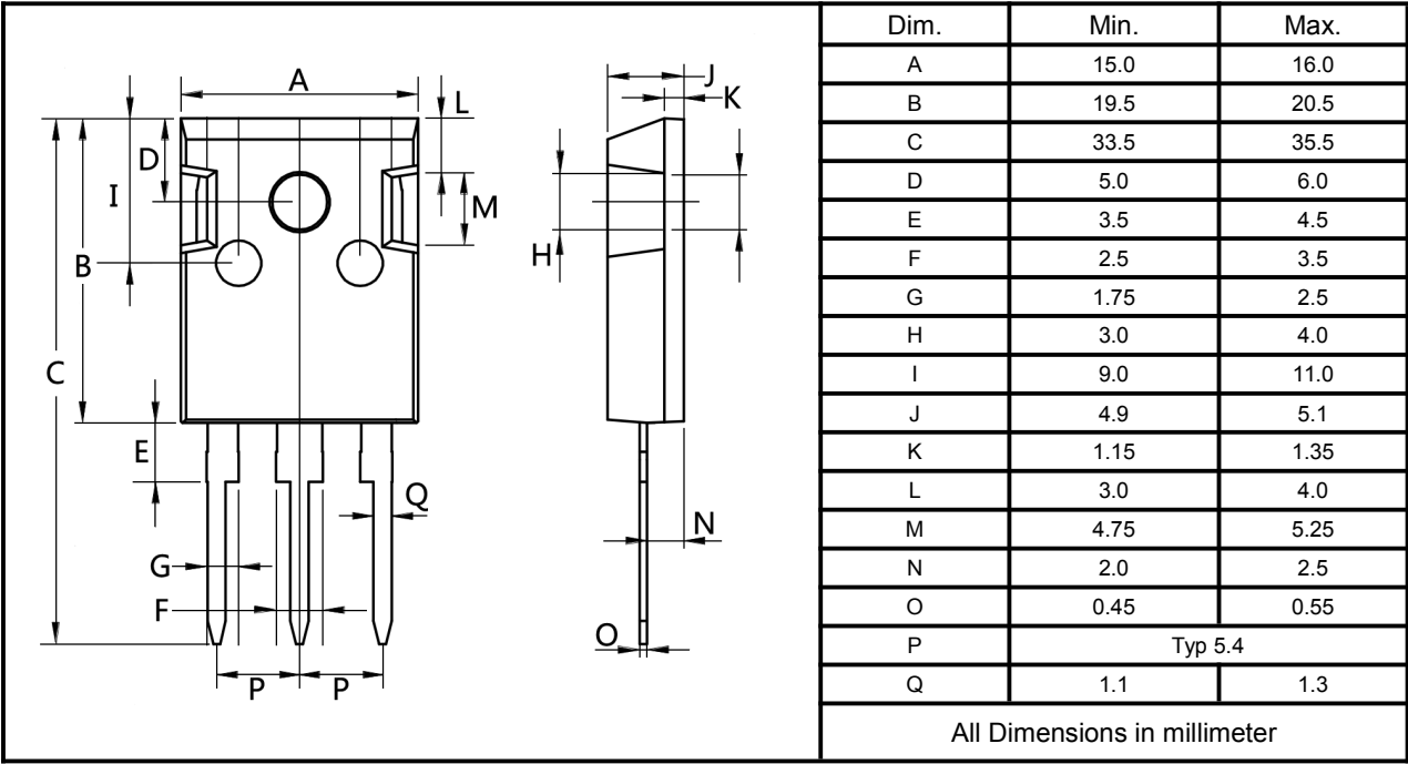
TO-247S 封装尺寸图
