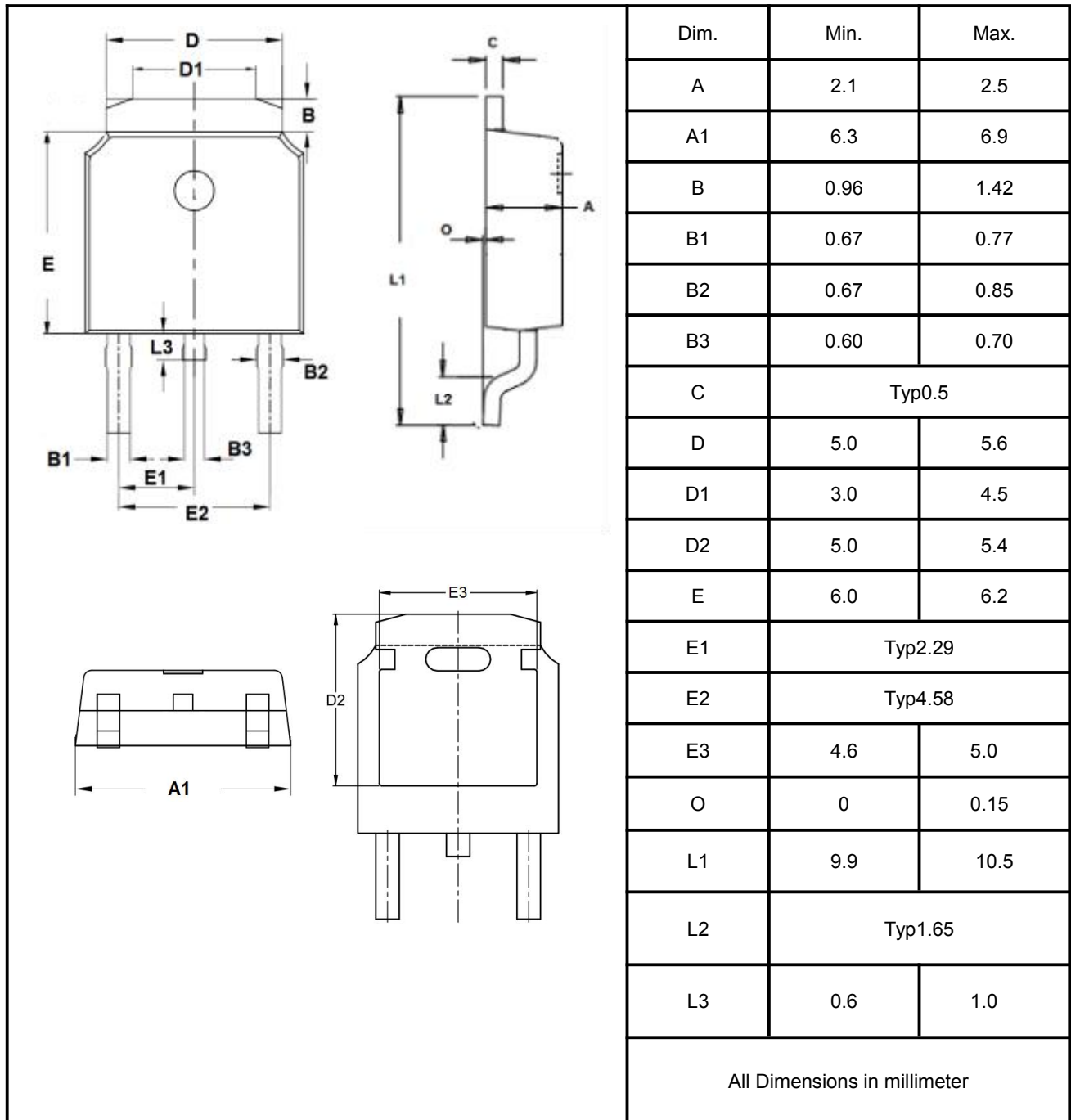
TO-252-6R 封装尺寸图
